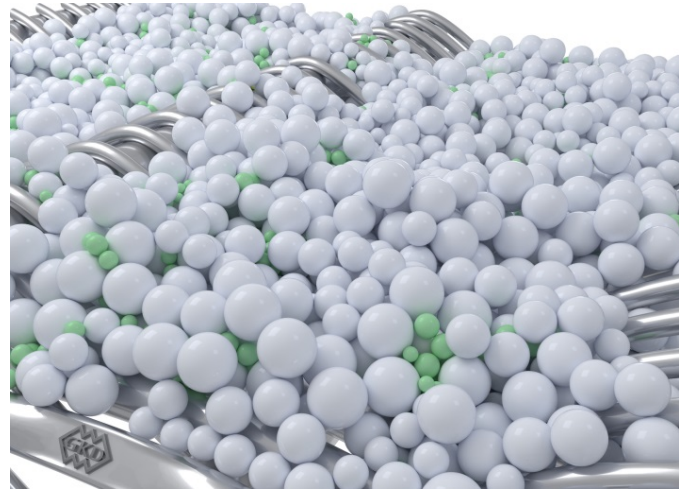
Bild 2: Unerreicht im Verhältnis von Porenöffnung zu Permeabilität ist die dreidimensionale Bindung der Porometric-Gewebe von GKD mit Trennschärfen von 20 bis 170 \mu\text{m} .
