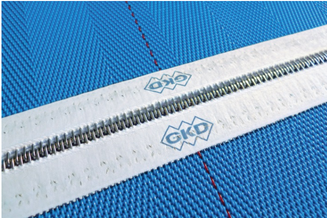
Bild 1: In Siebbandpressen punktet der Bandtyp 1003 von GKD bei den hohen auf ihn einwirkenden Belastungen durch seine außergewöhnliche Querstabilität und die besonders flache, robuste PAD-Naht.
