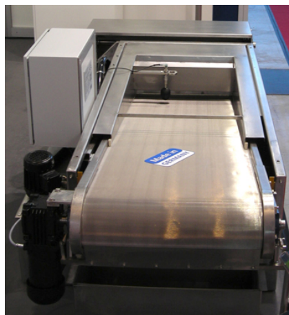
Bild 5: Bandfilter für die Partikeltrennung ab 40 µm.
